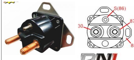
RELE AUXILIAR DE PARTIDA FORD 12V
